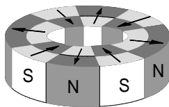
Abbildung 5: Magnetisierung radial
