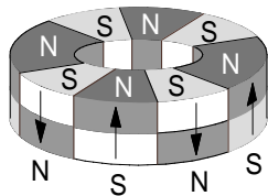
Abbildung 3: Magnetisierung axial
