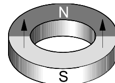
Abbildung 6: Magnetisierung diametral
