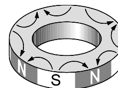
Abbildung 8: Magnetisierung außen lateral
