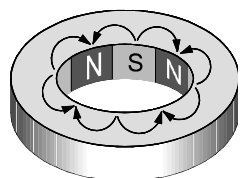
Abbildung 7: Magnetisierung innen lateral
